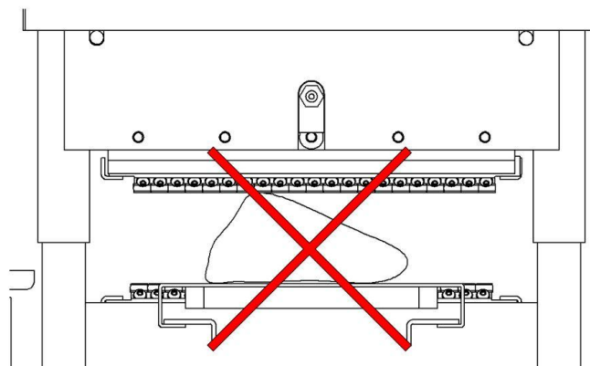
Abbildung 2.4-1: Maximale Abweichung Stein.
