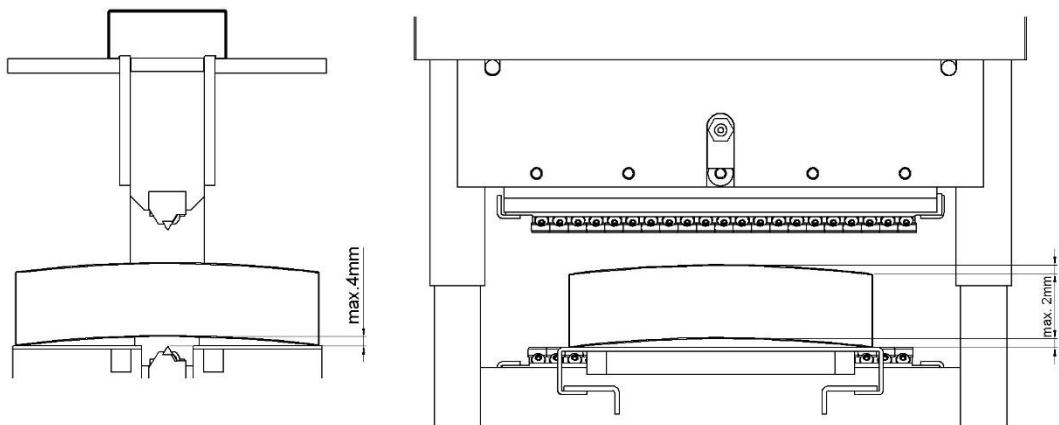
Abbildung 2.4-1: Maximale Abweichung Stein.
