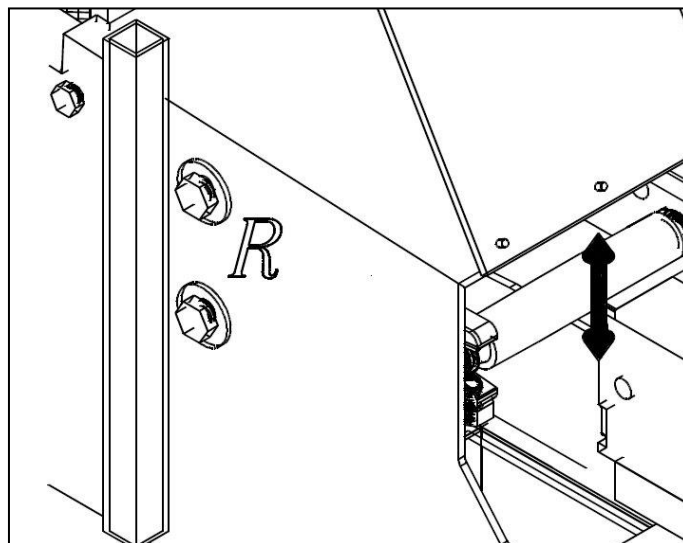
Figuur 4.6-4: Afstelling harthoogte slijprol
