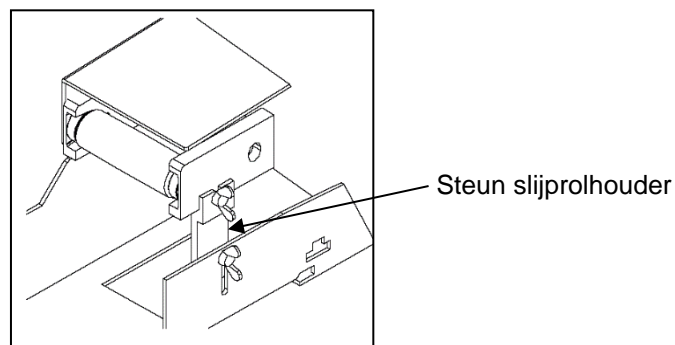
Figuur 4.6-2: Steun slijprolhouder
