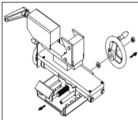
Figuur 4.6-6: Demonteren handwiel en spindel
