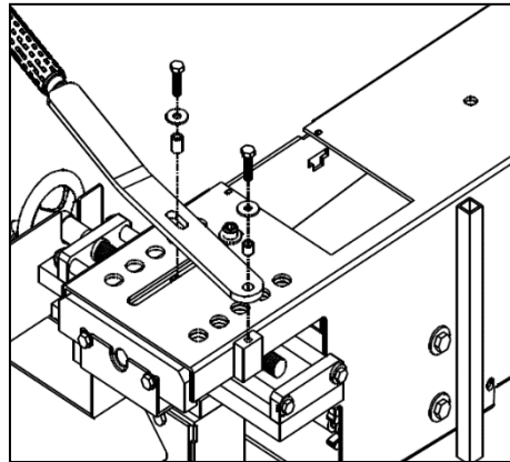
Figuur 4.6-7: Monteren hendel
