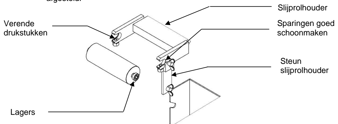
Figuur 4.6-4: Verwisselen slijprol
