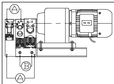
Figuur 7.3-1: Vervangen snijdoorn en/of veer 1 (weergegeven is machine AL1-2U)
