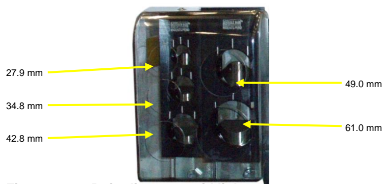
Figuur 4.6-1: Buis-diameters uitklinken
