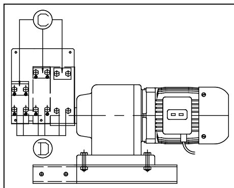
Figuur 7.3-2: Vervangen snijdoorn en/of veer 2 (weergegeven is machine AL1-2U)
