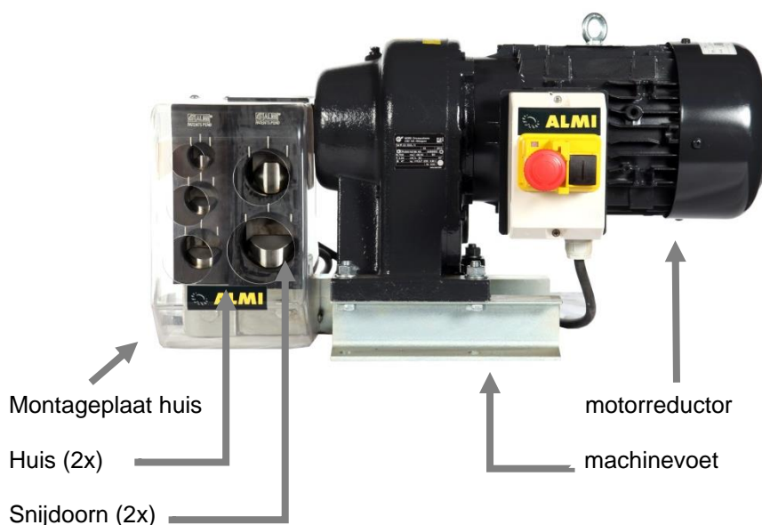
Figuur 4.2-1: Opbouw van de machine
