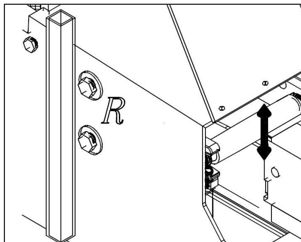
Figuur 4.6-5: Afstelling harthoogte slijprol
