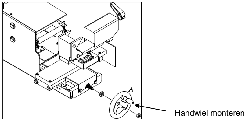
Figuur 0-2: Montage handwiel en hendel
