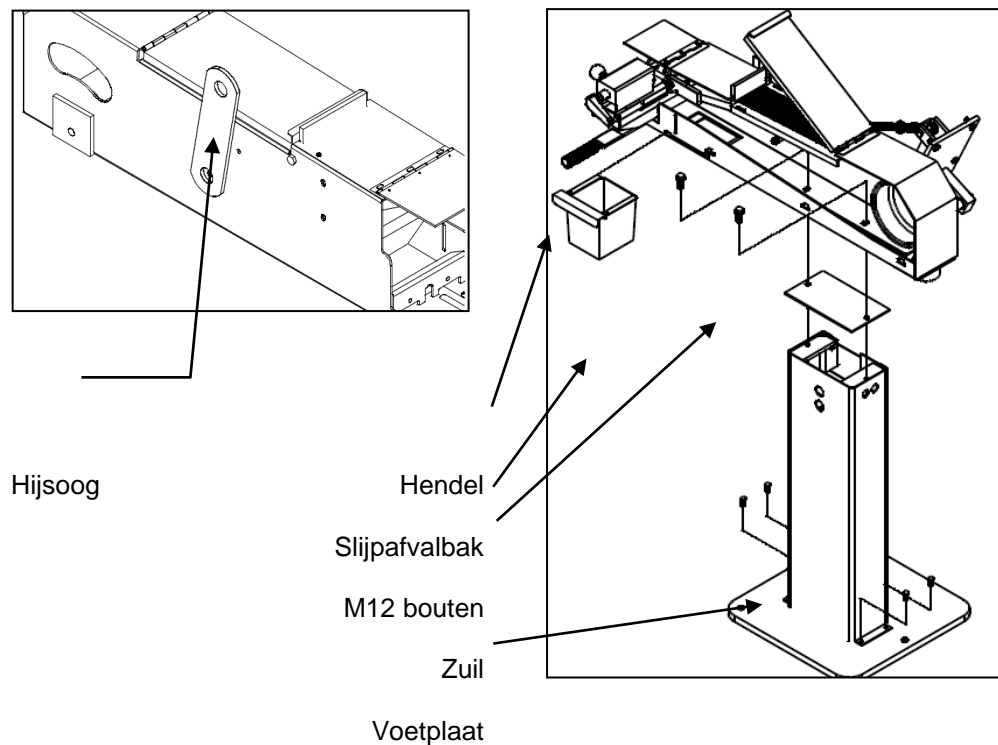
Figuur 0-1: Toelichting montage
