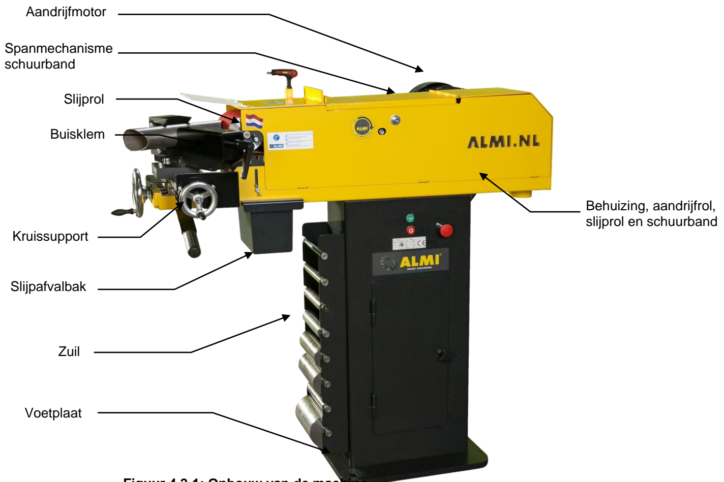
Figuur 4.2-1: Opbouw van de machine
