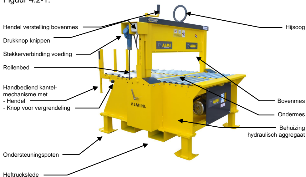
Figuur 4.2-1: Opbouw van de machine
